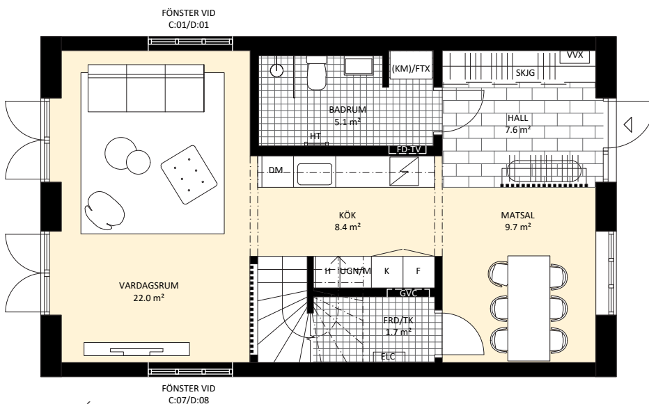
ENTRÉPLAN
